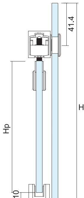
INSTALACIÓN RIEL SENCILLO A VIDRIO
