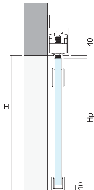
INSTALACIÓN RIEL SENCILLO A MURO
